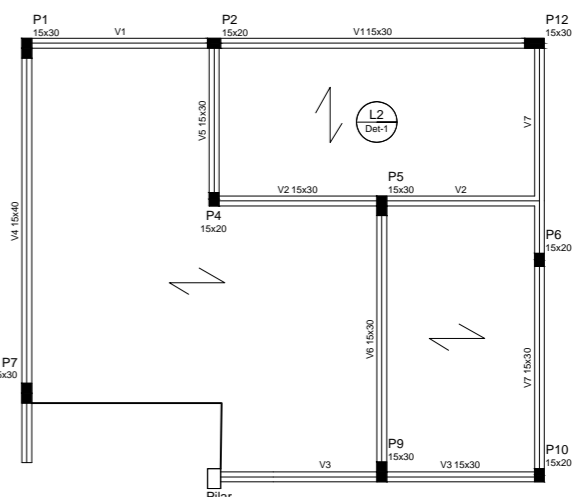
FÓRMAS CINTA SUPERIOR SALA 2
