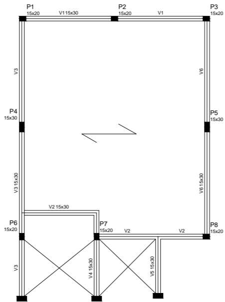
FÓRMAS CINTA SUPERIOR SALA 1 Esc. 1/
