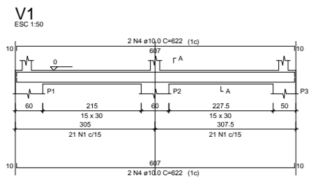
FÓRMAS BALDRAME SALA 1 Esc. 1/
