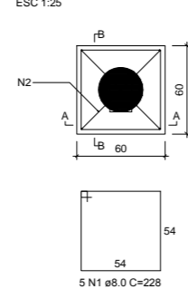
Bases 1x1C30 PLANTA ESC. 1:25
