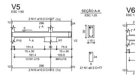
VIGAS BALDRAME SALA 1 Esc. 1/
