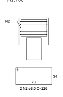
CORTE B-B ESC. 1:25
