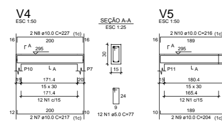
VIGAS CINTA SUPERIOR SALA 1 Esc. 1/
