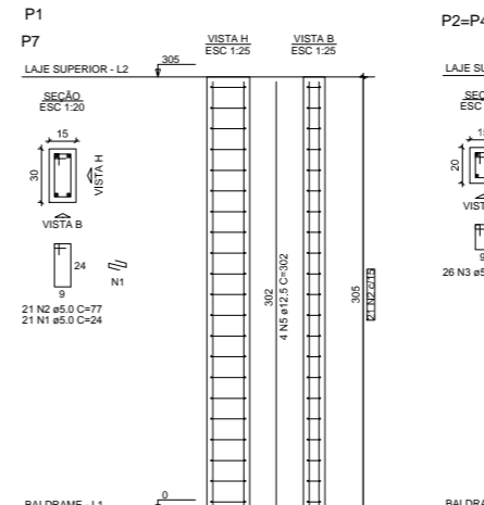
PILARES SALA 2 Esc. 1/
