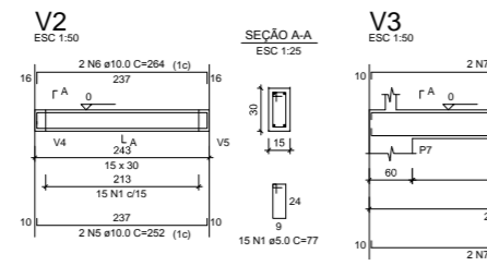
FÓRMAS CINTA SUPERIOR SALA 1 Esc. 1/
