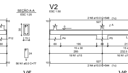
FÓRMAS BALDRAME SALA 2 Esc. 1/
