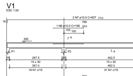
VIGAS BALDRAME SALA 2 Esc. 1/
