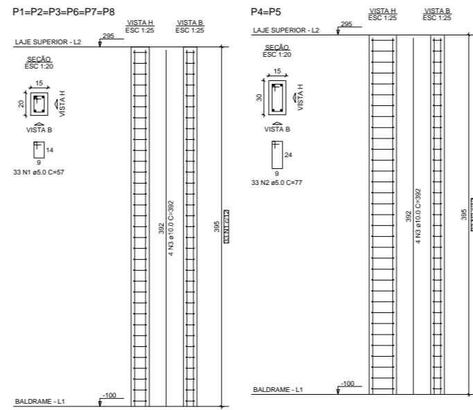
PILARES SALA 1 Esc. 1/
