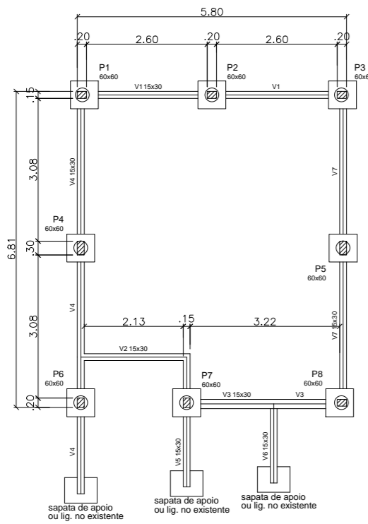
FÓRMAS BALDRAME SALA 1 Esc. 1/
