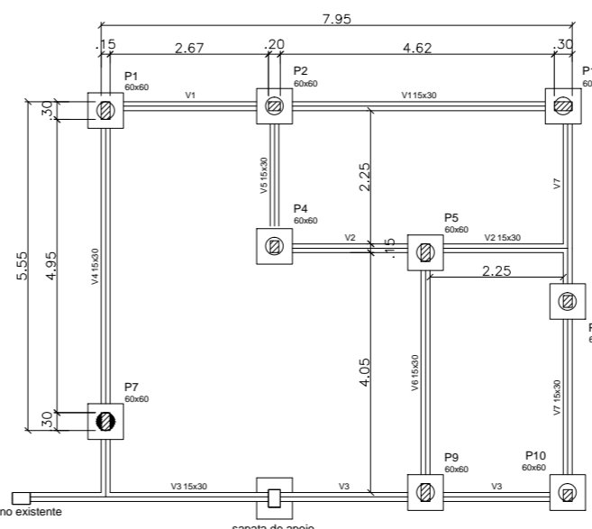
FÓRMAS BALDRAME SALA 2 Esc. 1/
