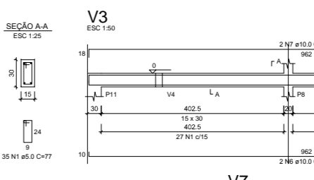
FÓRMAS CINTA SUPERIOR SALA 2
